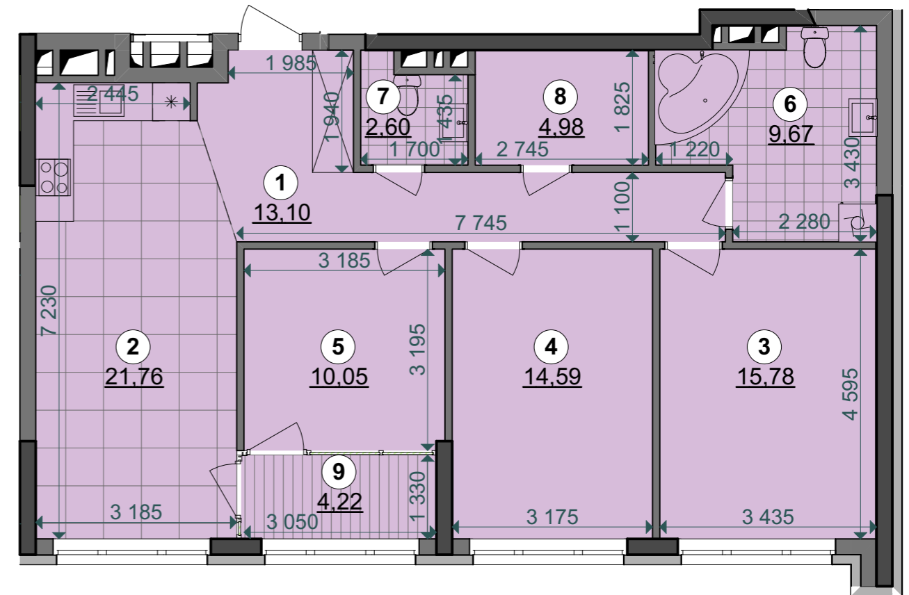
План квартири без перегородок
