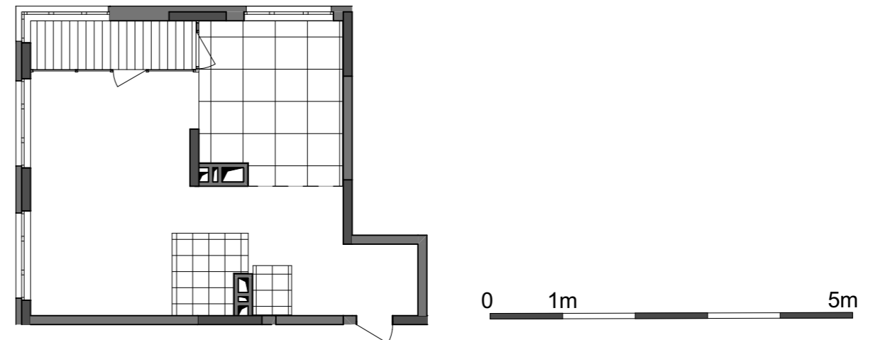
План квартири без перегородок
