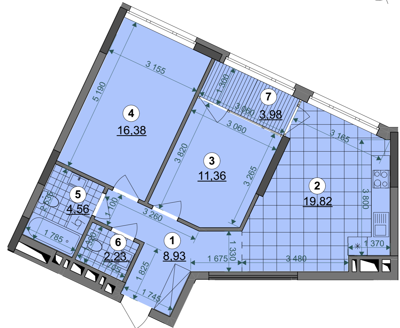
План квартири без перегородок
