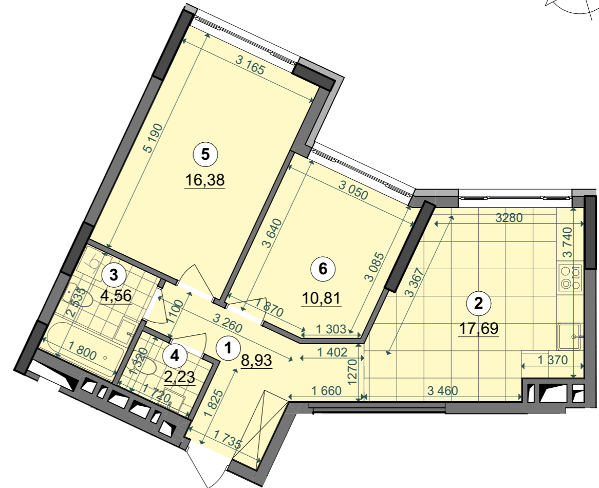
План квартири без перегородок
